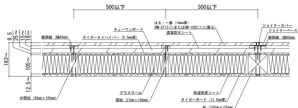
水平断面图
